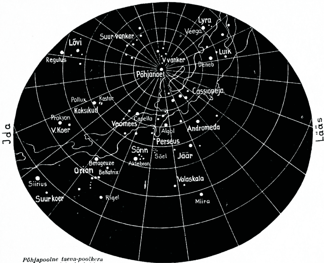
Põhjapoolne taeva-poolkera nagu ta on det. keskel kell 9 ö. ja det. lõpul kell 8 ö.
